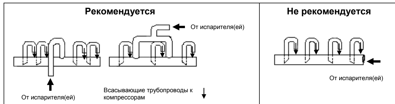
Рис. 6: Коллектор всасывания - рекомендации
